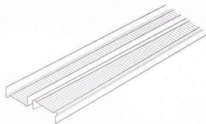
Khung thép mạ kẽm dùng cho trần chìm (C- Line)
